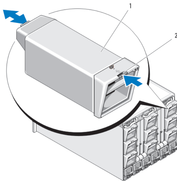
Abbildung 44. Lüftermodul entfernen und installieren
