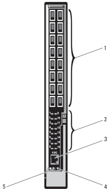
Abbildung 22. Infiniband-Switch-E/A-Modul Mellanox M4001F/M4001Q/M4001T
