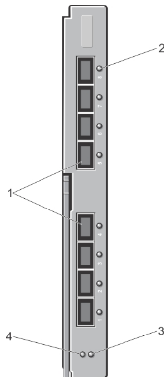
Abbildung 19. Cisco Nexus B22 Fabric Extender-Modul
