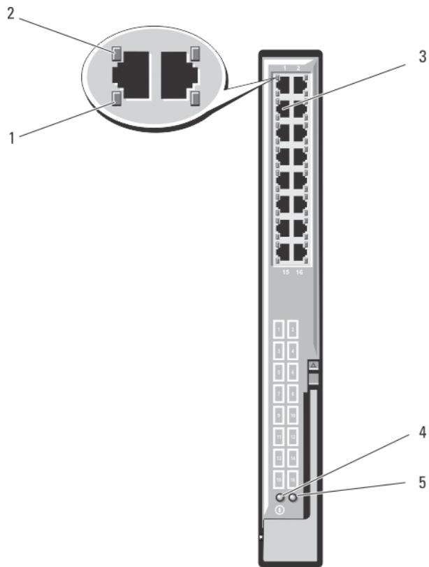
Abbildung 36. 10/100/1000-Mbit-Ethernet-Passthrough-E/A-Modul
