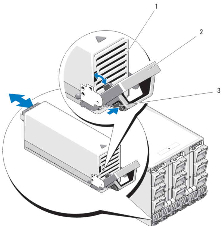
Abbildung 40. Netzteilmodul entfernen und installieren
