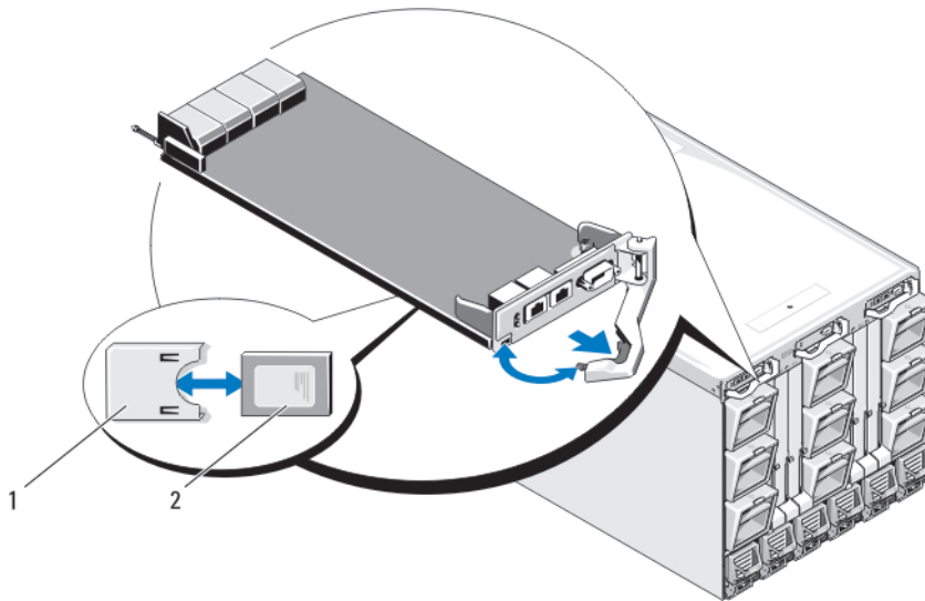
Abbildung 46. SD-Karte im CMC-Modul installieren
