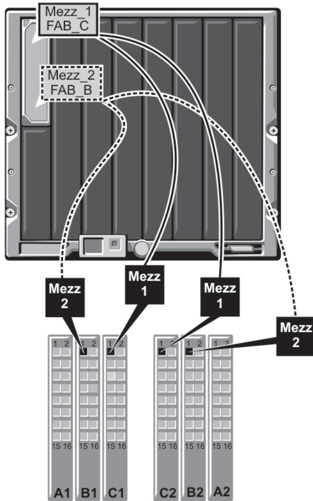
Abbildung 17. Beispiel für Portzuordnungen bei einem Blade mit halber Bauhöhe
