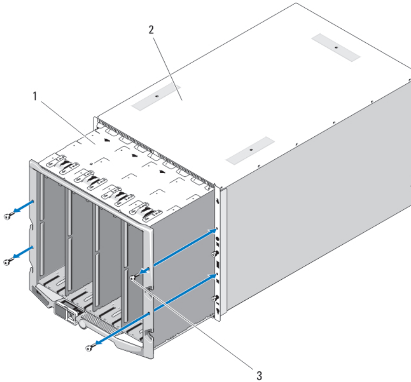
Abbildung 50. Vordere Modulträgerbaugruppe entfernen und installieren
