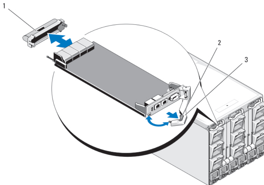
Abbildung 45. CMC-Modul oder iKVM-Modul entfernen und installieren (CMC-Modul dargestellt)
