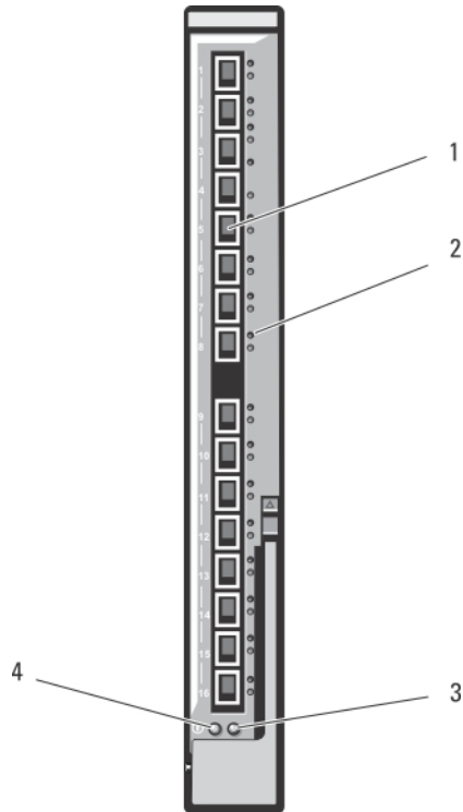
Abbildung 34. KR-Passthrough-E/A-Modul Dell 10 GbE
