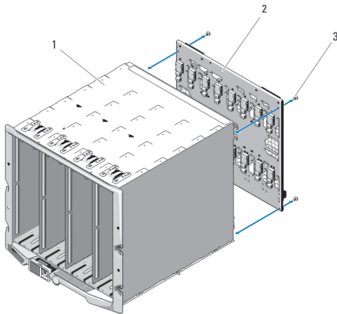
Abbildung 51. Mittelplatine entfernen und installieren
