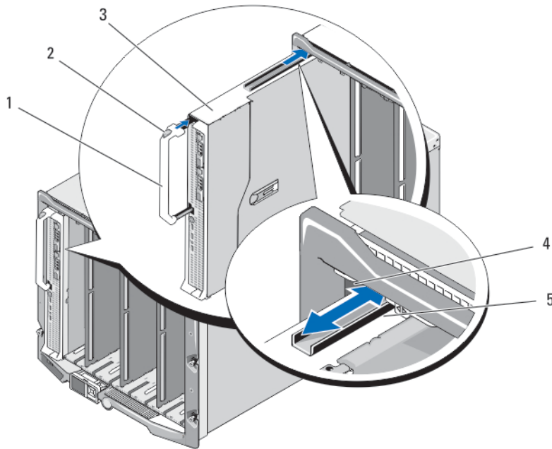
Abbildung 38. Blade mit voller Bauhöhe entfernen und installieren
