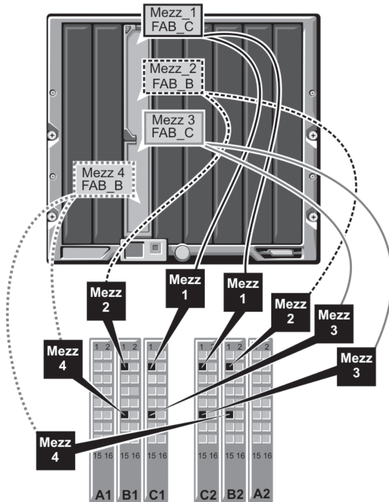
Abbildung 16. Beispiel für die Portzuordnung bei einem Blade mit voller Bauhöhe – Blade 3 (gilt nicht für PowerEdge M610x)
