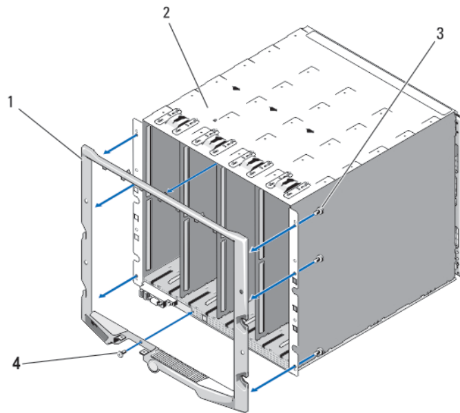
Abbildung 49. Frontverkleidung entfernen und anbringen
