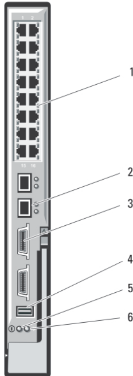
Abbildung 28. 1-Gbit-Ethernet-Switch-E/A-Modul PowerConnect M6348
