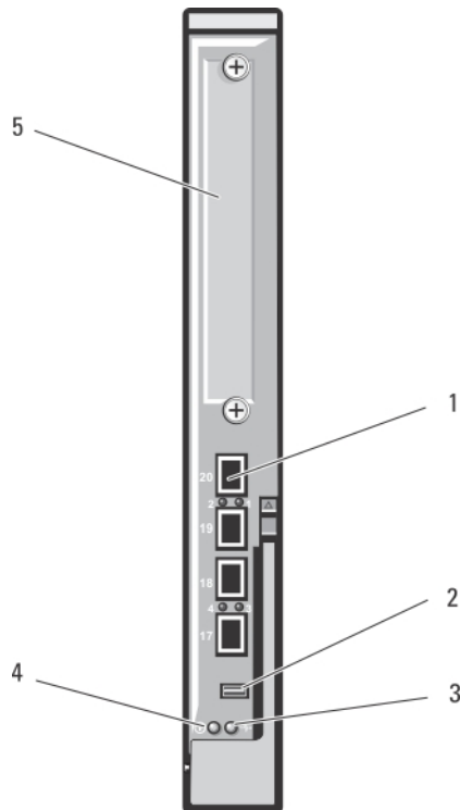
Abbildung 23. Dell PowerConnect-KR 8024-k Switch
