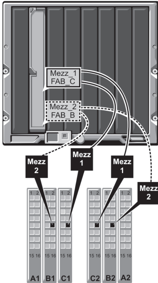
Abbildung 15. Beispiel einer Portzuordnung bei PowerEdge M610x – Blade 2
