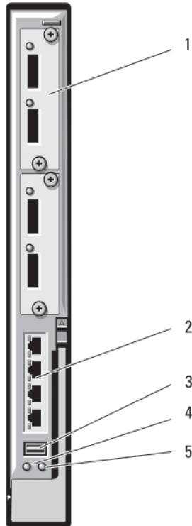
Abbildung 29. Ethernet-Switch-E/A-Modul PowerConnect M6220
