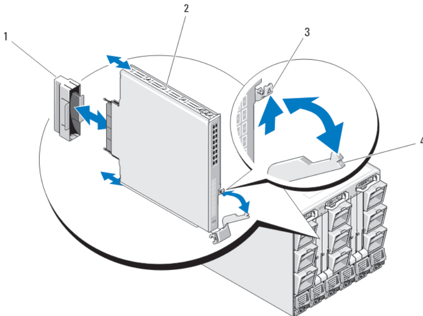
Abbildung 48. E/A-Modul entfernen und installieren
