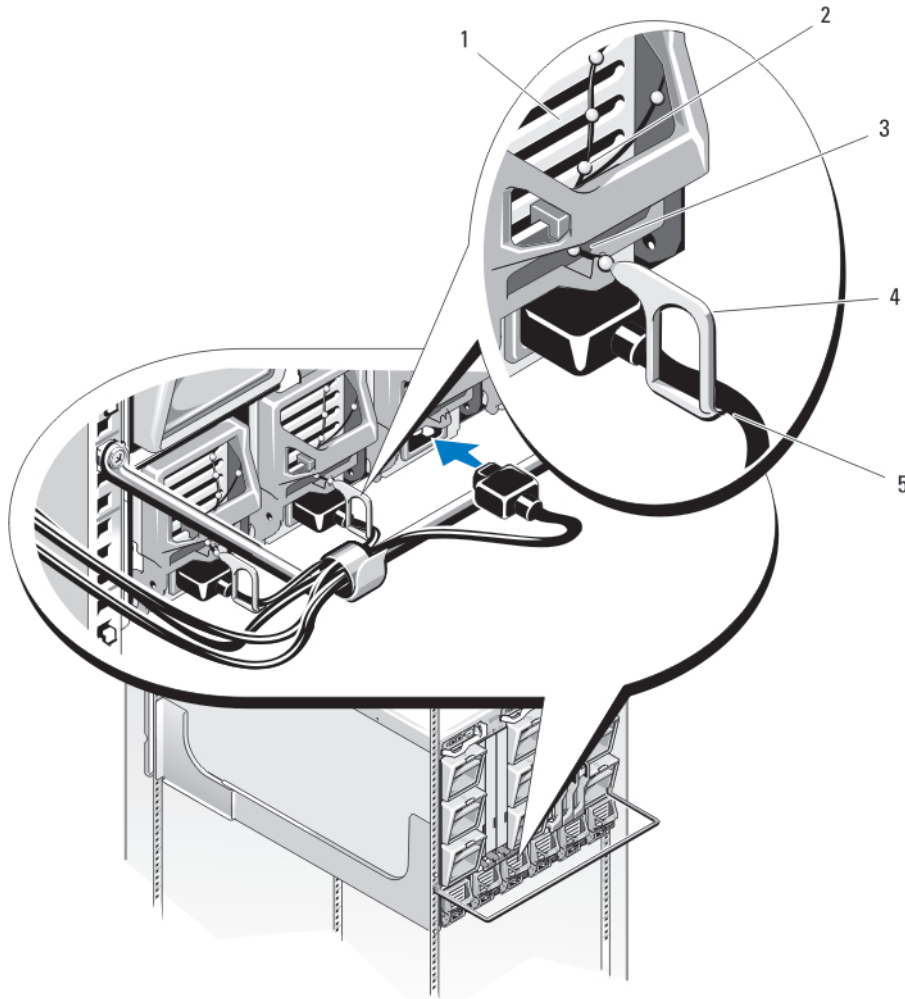
Abbildung 39. Halteklemme für das Stromkabel
