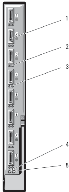
Abbildung 25. DDR-Infiniband-Switch-Modul Mellanox M2401G
