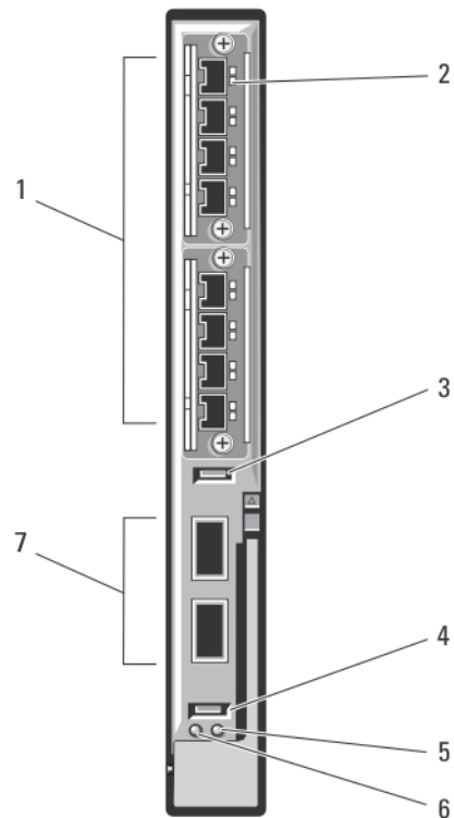
Abbildung 21. 10/40-GbE-Switch-E/A-Modul Dell Force10 MXL
