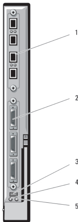
Abbildung 30. 10-Gbit-Ethernet-Switch-E/A-Modul PowerConnect M8024
