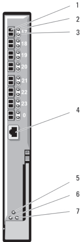
Abbildung 32. E/A-Modul Brocade M5424 FC8
